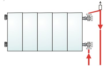
подключение одностороннее, справа (макс. 5 коллекторов)
